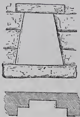
Élévation et plan de niches à Ollantaïtambo.
